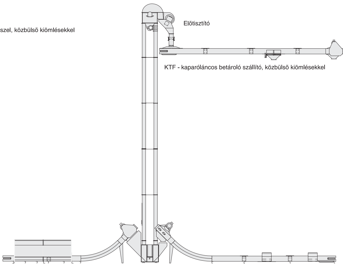
KTG - garat szállító felszíni töltőgarattal
